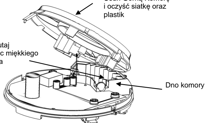
Rysunek 2 – Usunięcie obudowy zewnętrznej odsłania komorę optyczną.
