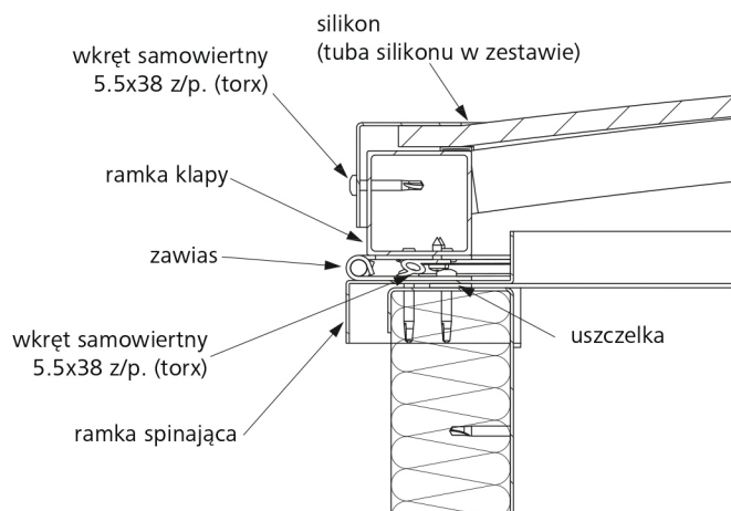
Mocowania kopułki do podstawy klapy
