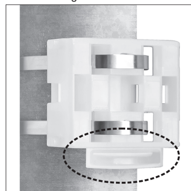
Montaż na maszcie / Mast mounting
